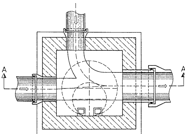
Grundriß
