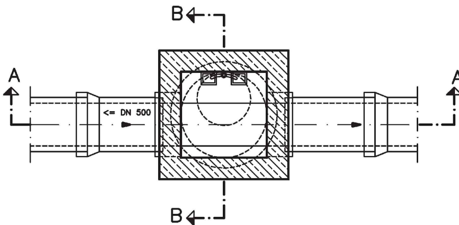
Grundriss
