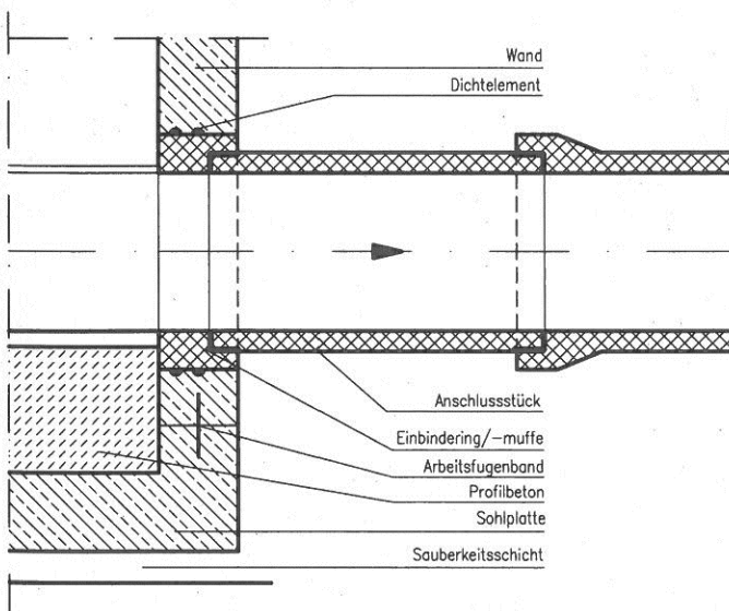
Anschluss von Beton- und Stahlbetonrohren mit Einbinder
