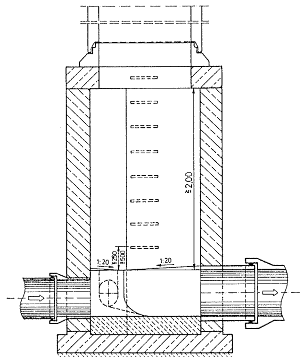
Schnitt A-A
