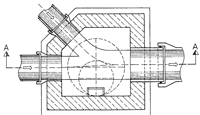
Grundriß
