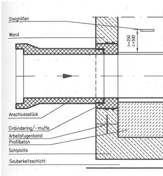
Anschluss von Beton- und Stahlbetonrohren mit Einbinder
