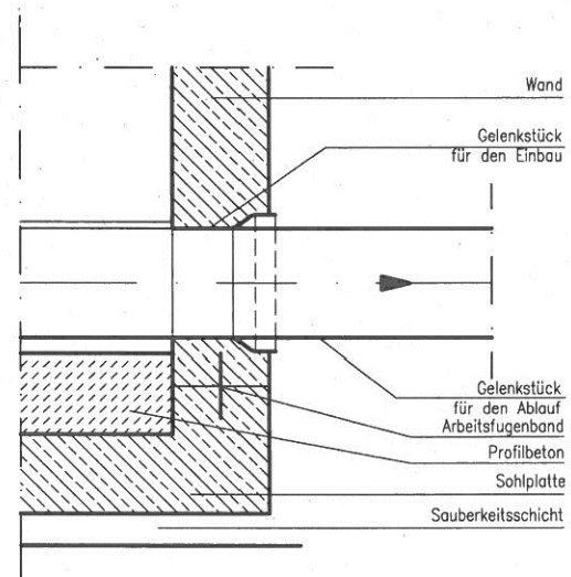
Anschluss von Steinzeugrohren
